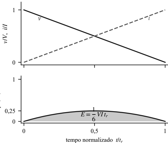
(a) carga resistiva
