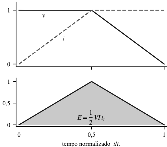
(b) carga inductiva grampeada
